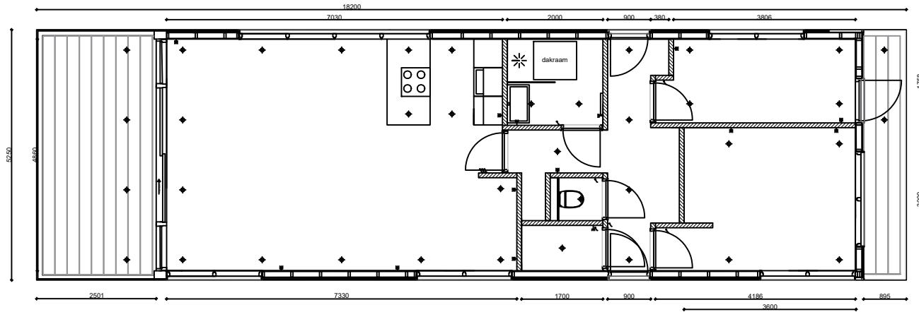
Plattegrond
