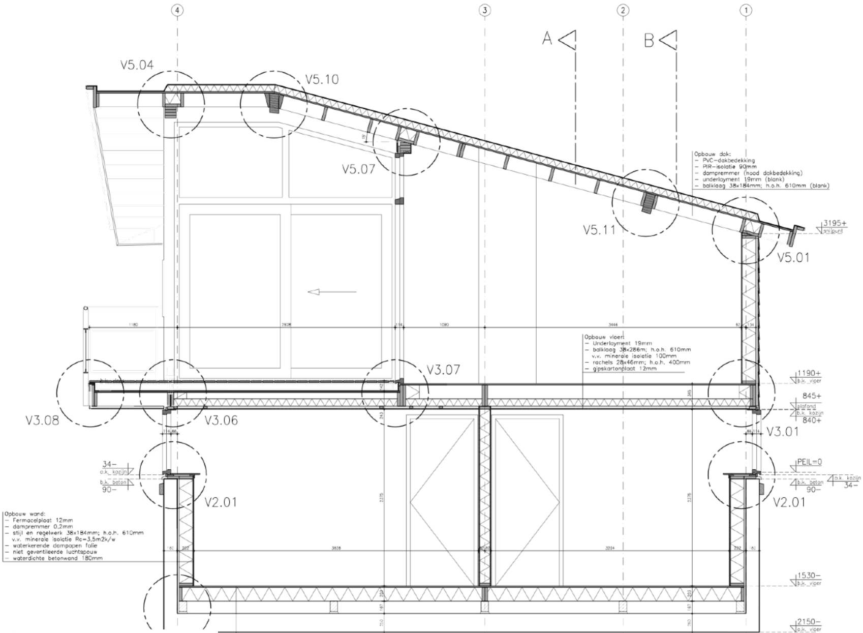
Technische Zeichnung Maas-Villa.
